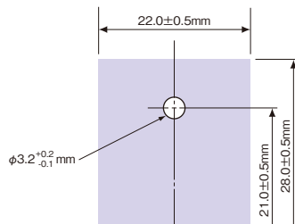
TO-3PL型 Model T0-3PL
