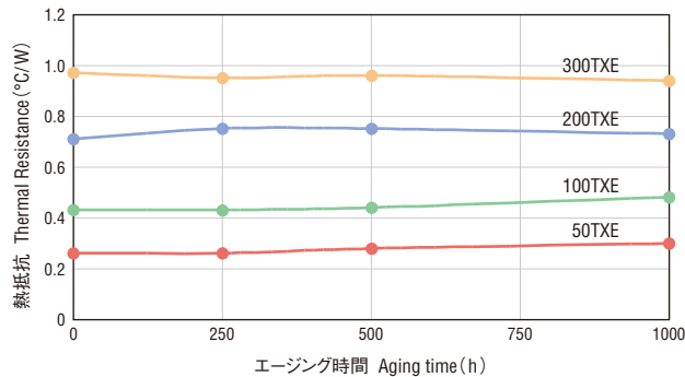
■ 熱抵抗変化 Thermal Resistance Change (85°C/85%RH)
