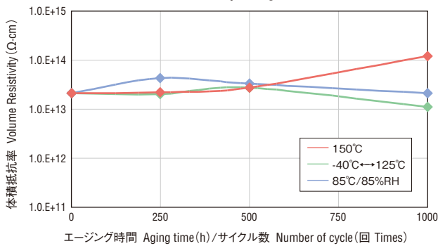
■ 体積抵抗率変化 Volume Resistivity Change
