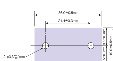
TO-3P2型 Model T0-3P2
