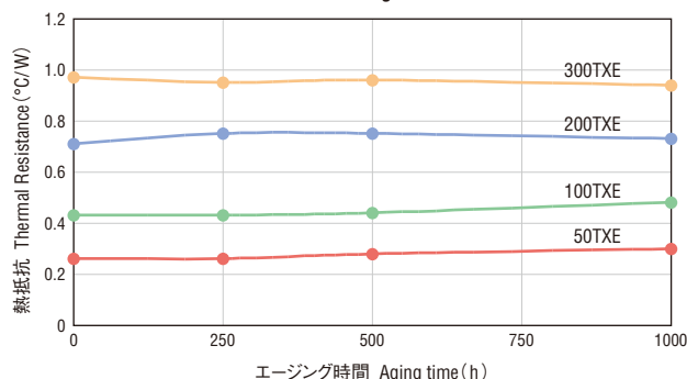
■ 熱抵抗変化 Thermal Resistance Change (150°C)
