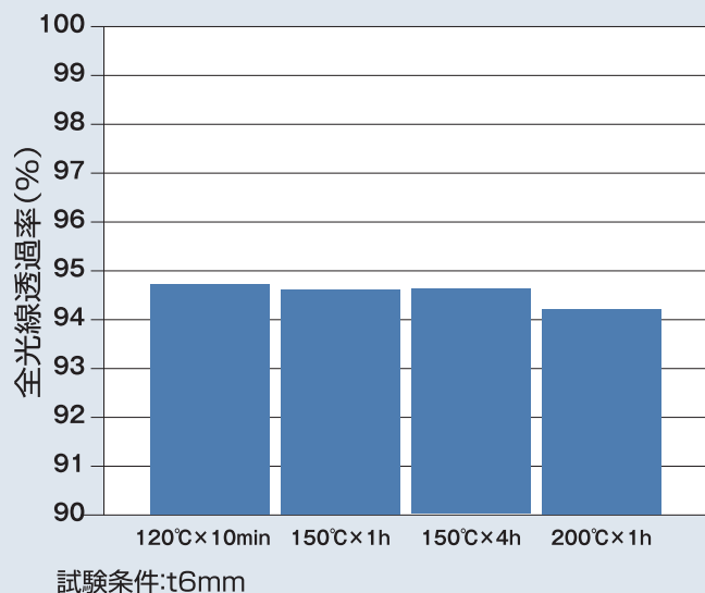
■ KE-2061-60-A/Bの全光線透過率
