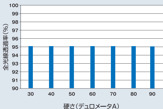
■ 硬さと全光線透過率
