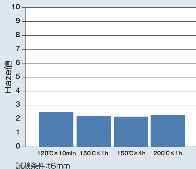
■ KE-2061-60-A/BのHaze値
