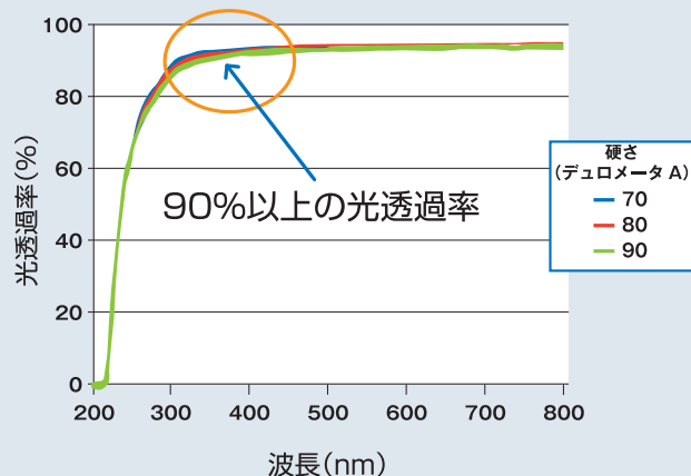
■ 波長と光透過率
