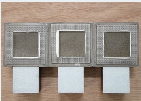
パッチシールクロスの破断状況
