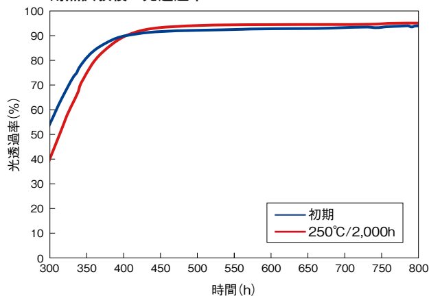
LEDデバイス用封止材 KER-2936-A/B 耐熱試験後の光透過率
