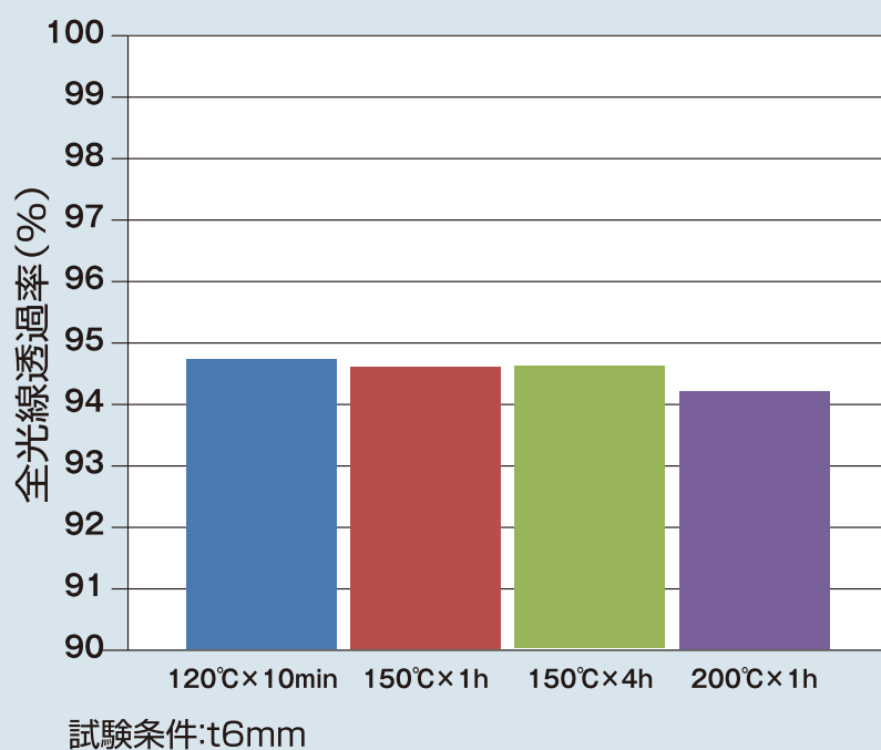
■ KE-2061-60-A/Bの全光線透過率
