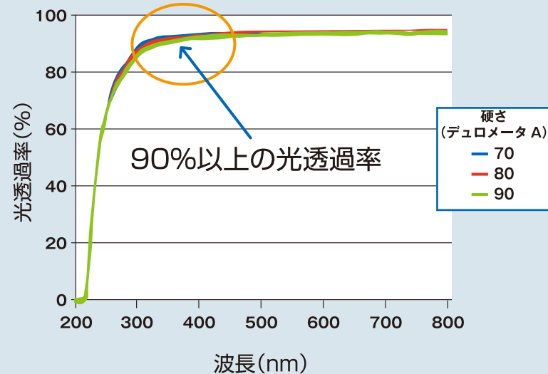
■ 波長と光透過率
