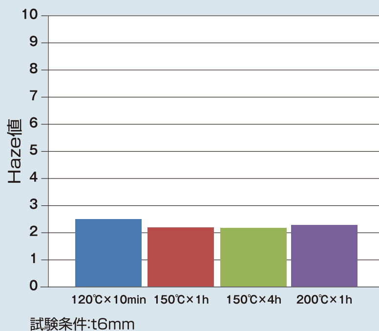
■ KE-2061-60-A/BのHaze値
