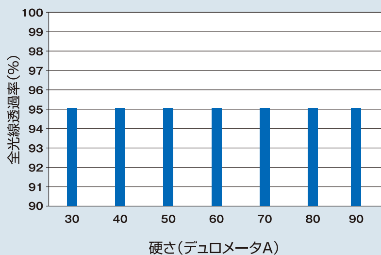
■ 硬さと全光線透過率
