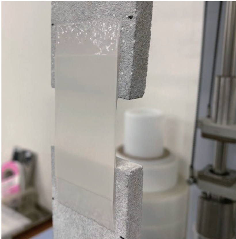
引張りせん断試験の様子
