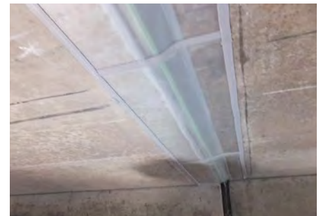
段差のある目地に施工した例
