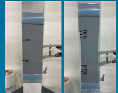
テープありではパッチシール端部を保持
